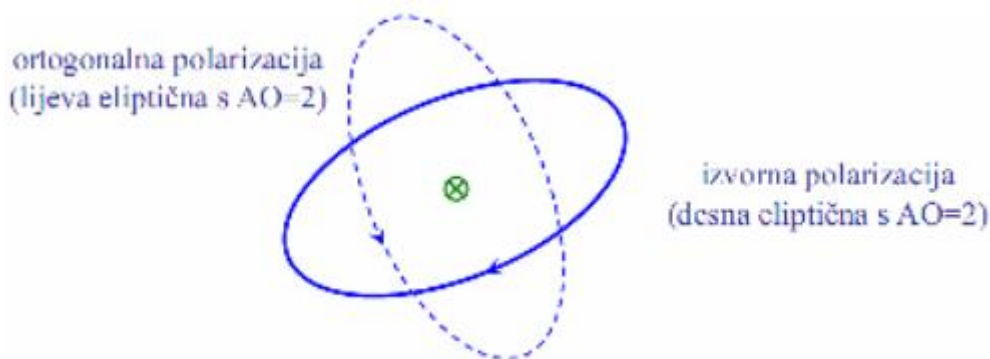
Slika 2.10 Ortogonalna polarizacija [1]
