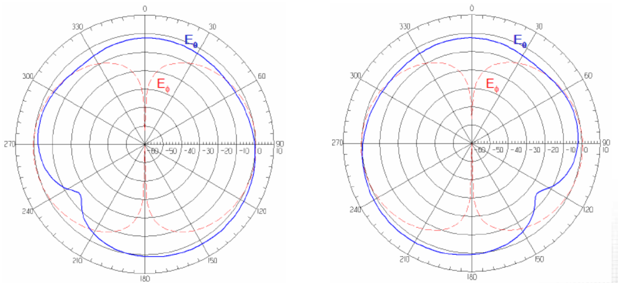
Slika 4.6 Dijagrami zračenja sustava s dvije antene [7]
