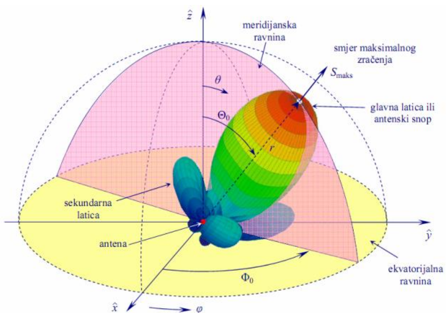
Slika 2.6 Prostorni dijagram zračenja antene Antena se nalazi u ishodištu cilindričnog koordinatnog sustava. Bojom je označena intenzitet zračenja (plavo \rightarrow crveno) [1]
