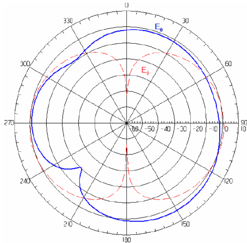
Slika 4.5 Dijagram zračenja [7]
