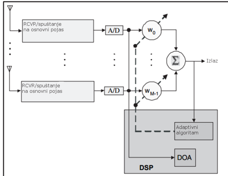
Slika 3.7 Blok dijagram sustava adaptivnog niza [5]
