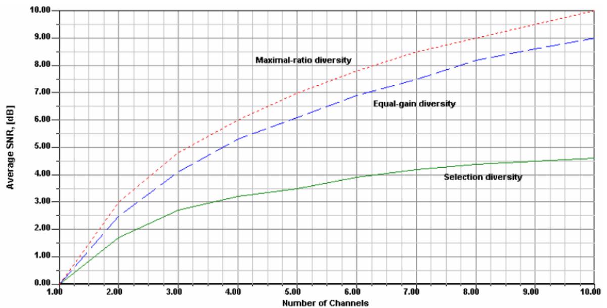
Slika 4.1 Odnos signala i šuma u odnosu na broj kanala [7]
