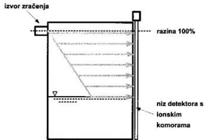
Slika 3.7.1 Radiometrijska metoda mjerenja razine.[2]
