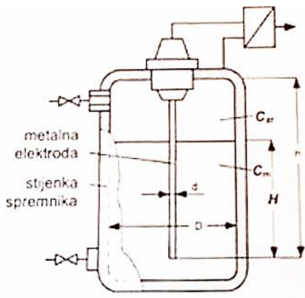
Slika 3.3.1 Mjerenje s uronjenom elektrodom. [2]
