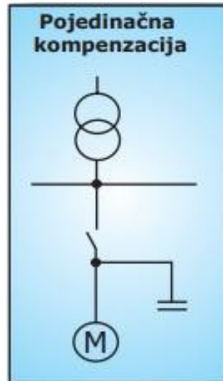
Slika 3.8. Shema pojedinačne kompenzacije [1]
