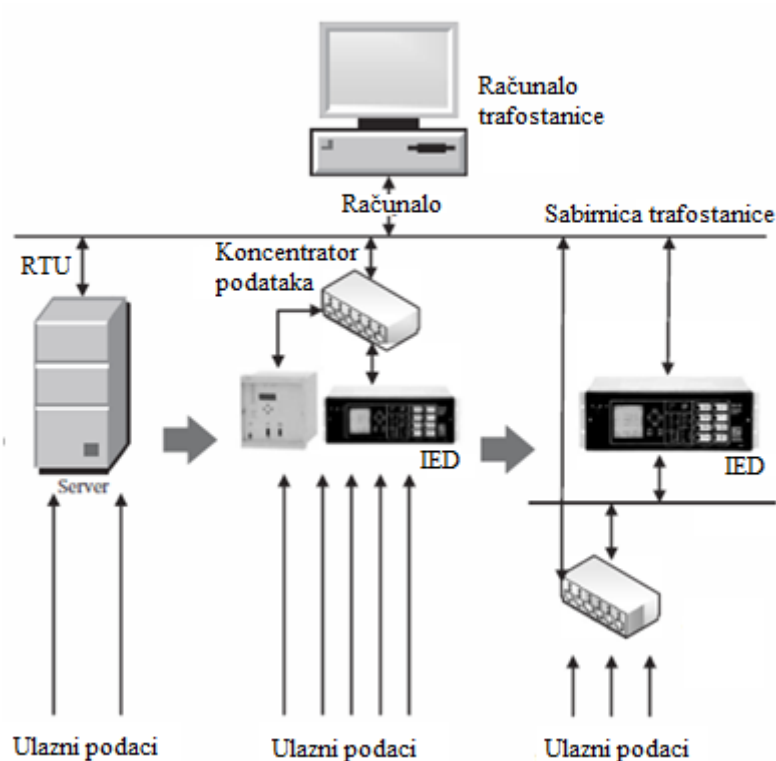
Slika 2.7. Razvoj SCADA sustava tijekom godina
