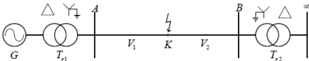
Slika 3.8. jednopolna shema promatranog sustava [8]
