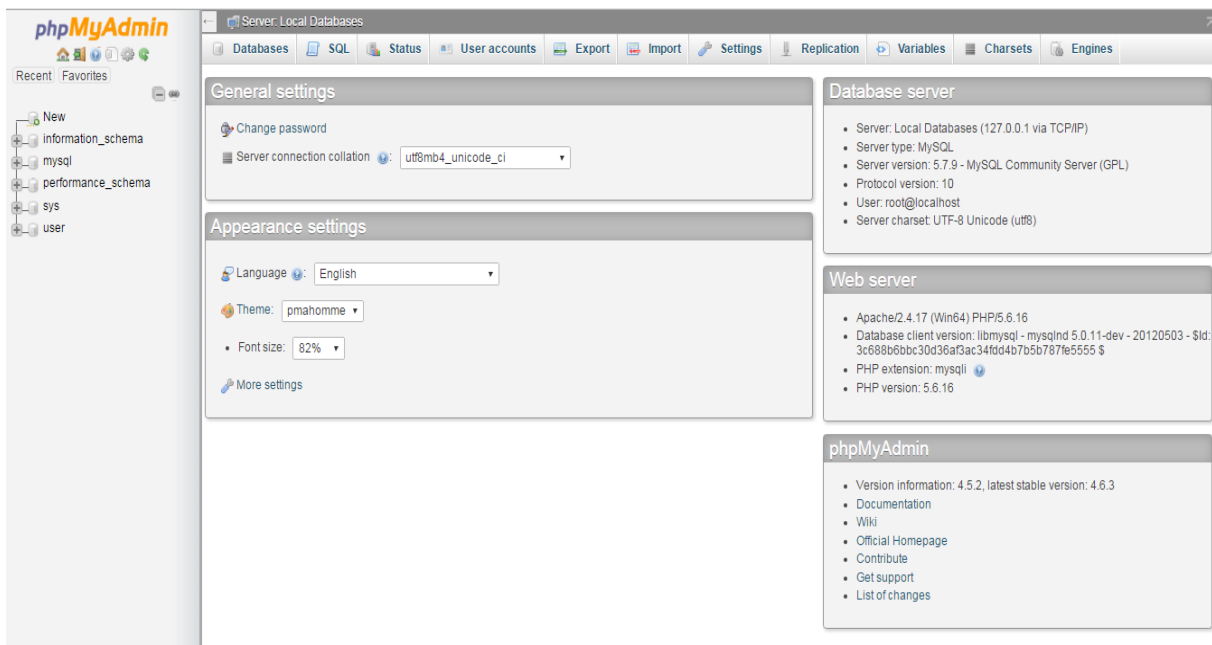
Sl. 2.4. phpMyAdmin
