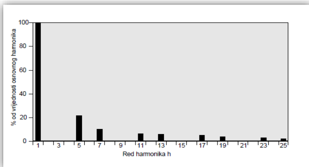
Slika 2.18. Harmonički spektar strujnog harmonika šestpulsnog mosta.
