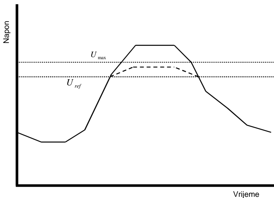
Grafikon 3.14. Utjecaj prenaponskog isključenja na vrijednost napona bez isključenja (puna linija) i sa isključenjem (iscrtkana linija)
