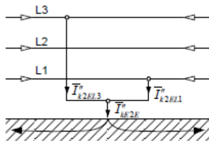
SI 2.5. Dvofazni kratki spoj uz dodir sa zemljom[2] SI. 2.6. Jednofazni kratki spoj[2]
