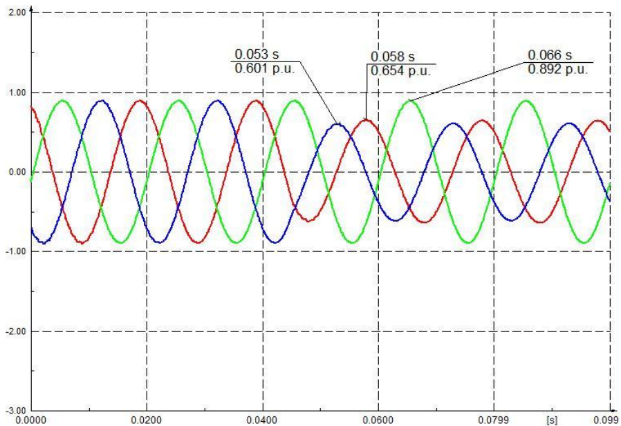
Sl. 3.38. Valni oblici napona pojedinih faza na sekundaru 20/0.4 kV za jednofazni kratki spoj
