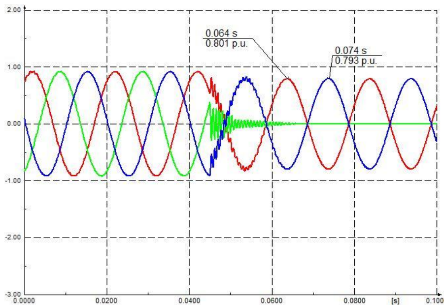
Sl. 3.22. Valni oblici napona pojedinih faza na sekundaru za dvofazni kratki spoj
