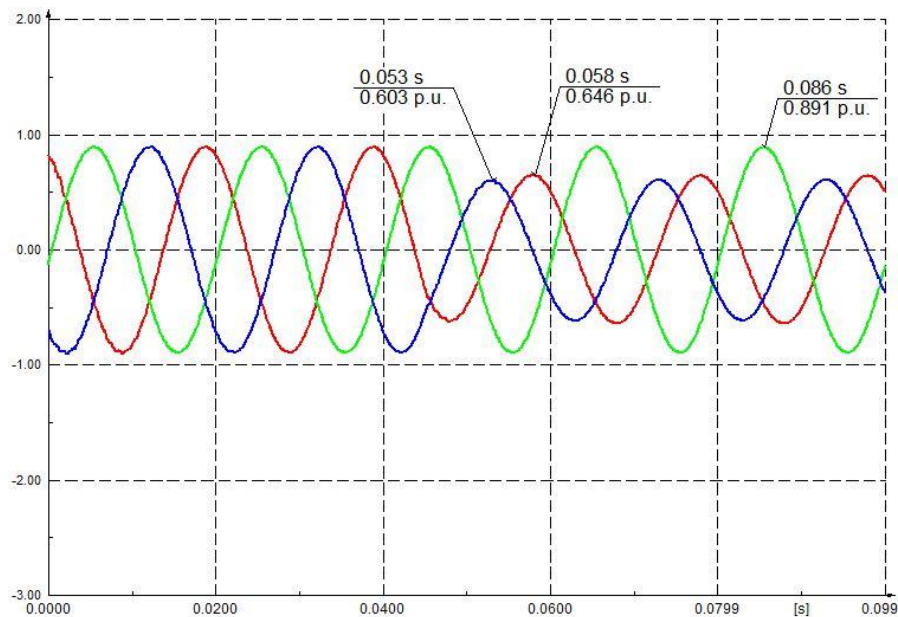
Sl. 3.31. Valni oblici napona pojedinih faza na sekundaru 20/0.4 kV za jednofazni kratki spoj
