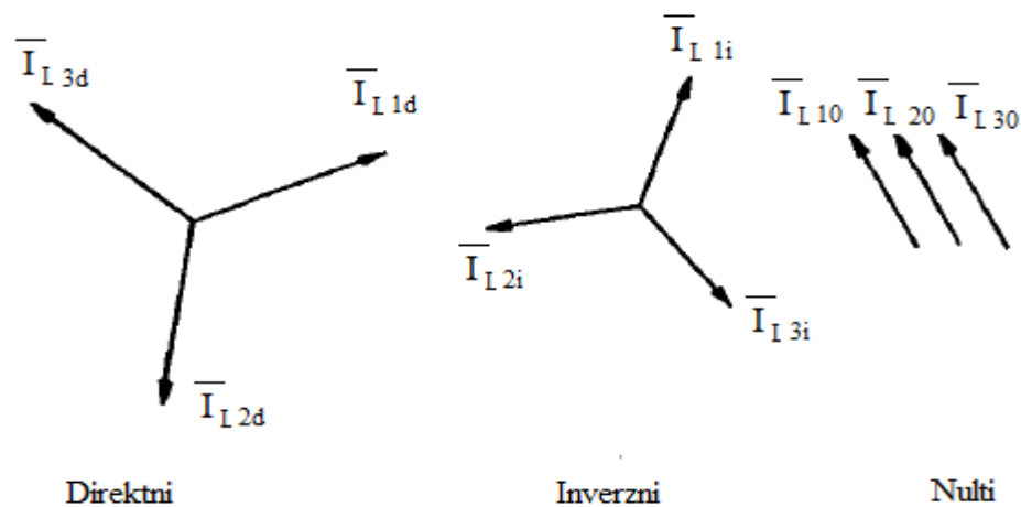
Sl. 2.10. Simetrične komponente
